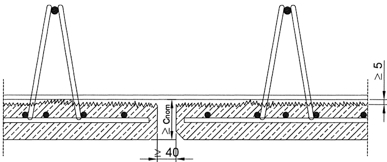
Bild 3: Druckfuge
