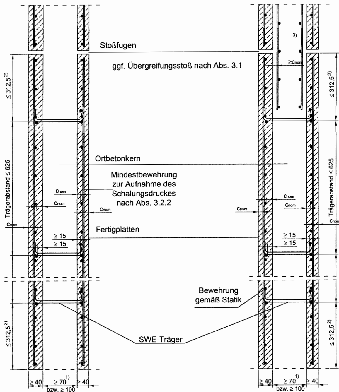
Bild 10: unbewehrte Wand
