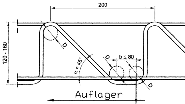
Bild 6: Filigran-EQ-Gitterträger
