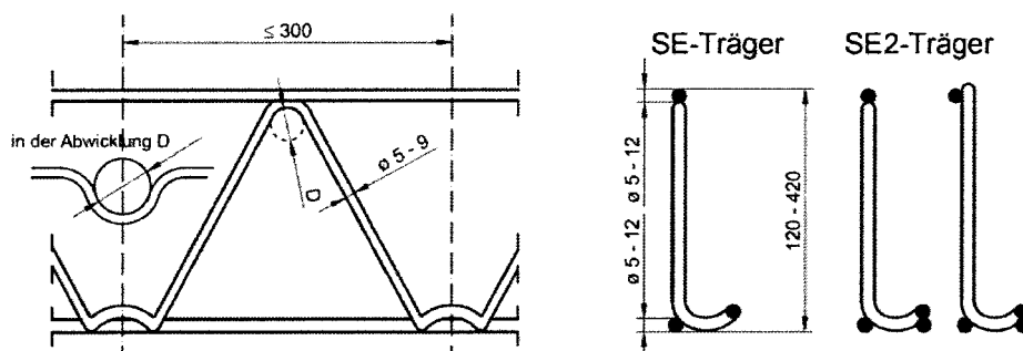
Bild 4: Filigran-SE/SE2-Gitterträger
