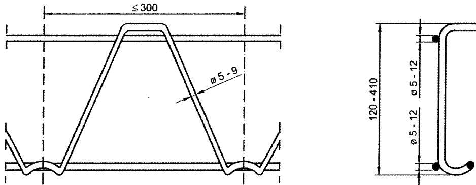
Bild 5: Filigran-SWE-Gitterträger
